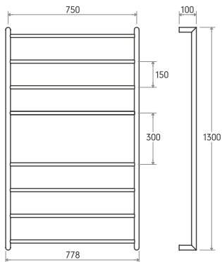
TLH6-130x75
