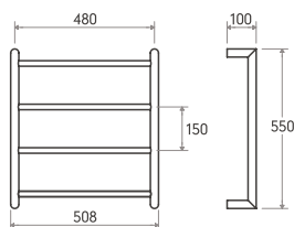
TLH5-55 x 48
