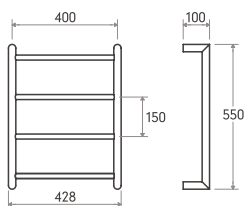
TLH5-55 x 40
