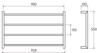
TLH5-55 x 90
