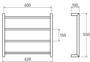
TLH5-55 x 60
