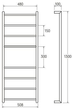
TLH6-130x48
