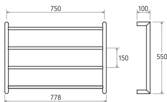
TLH5-55 x 75
