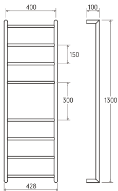
TLH6-130x40
