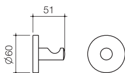
Liano Nexus Robe Hook 96125B
