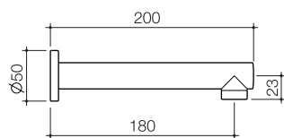
Liano Nexus Bath Outlet 96154B
